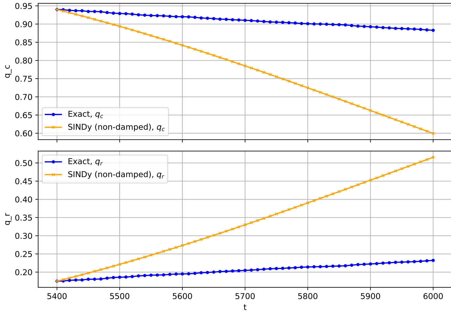
Trajectory No. 2449
