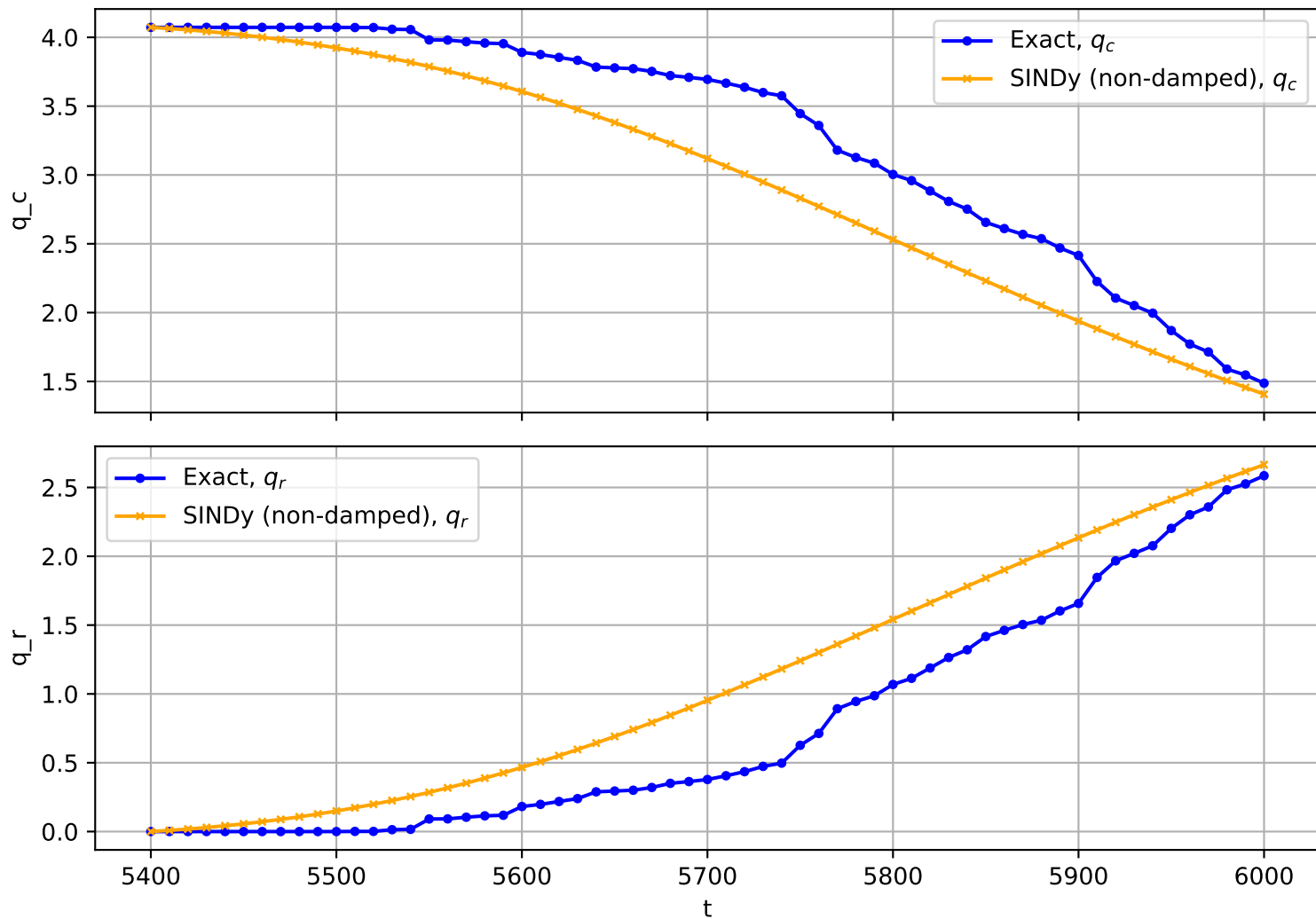
Trajectory No. 2497
