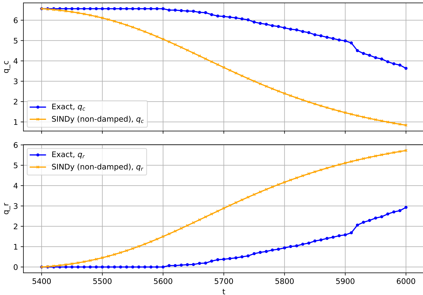
Trajectory No. 2506
