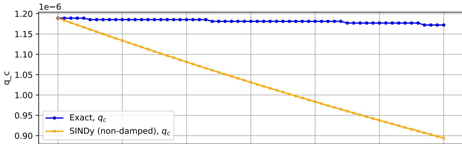
Trajectory No. 2548
