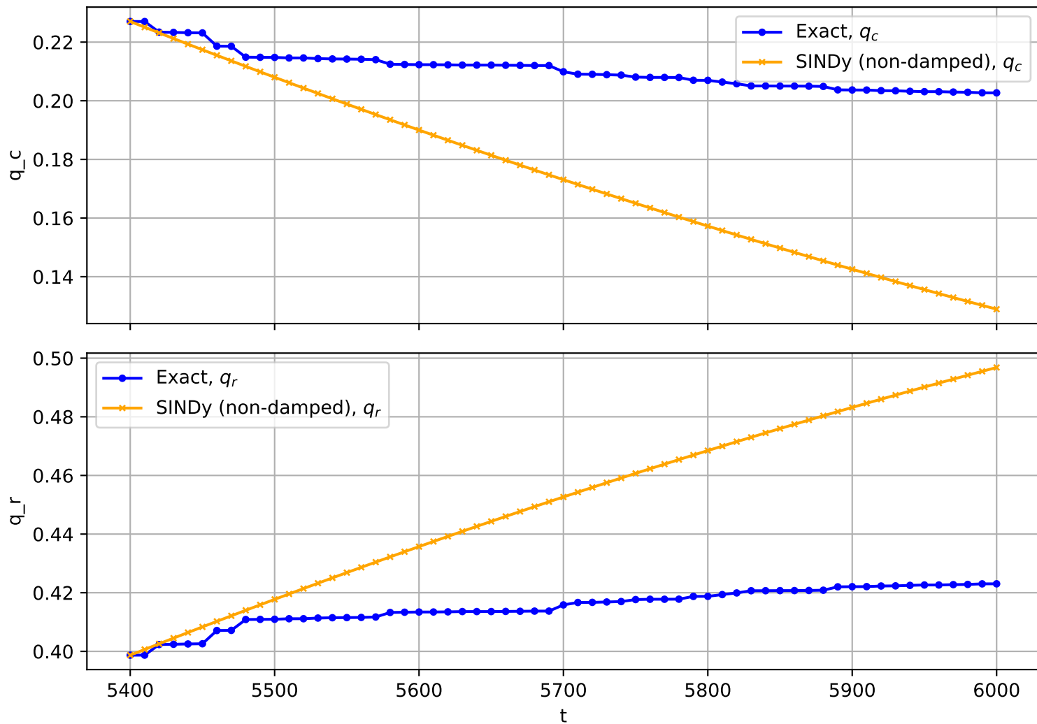
Trajectory No. 2551
