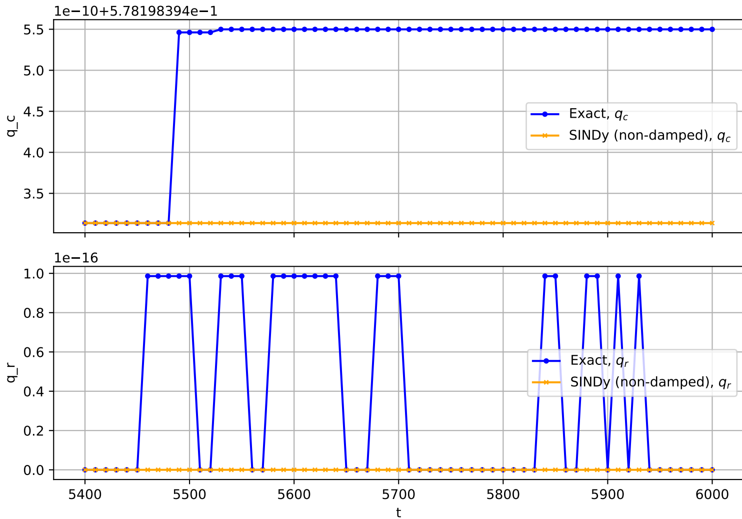
Trajectory No. 2553
