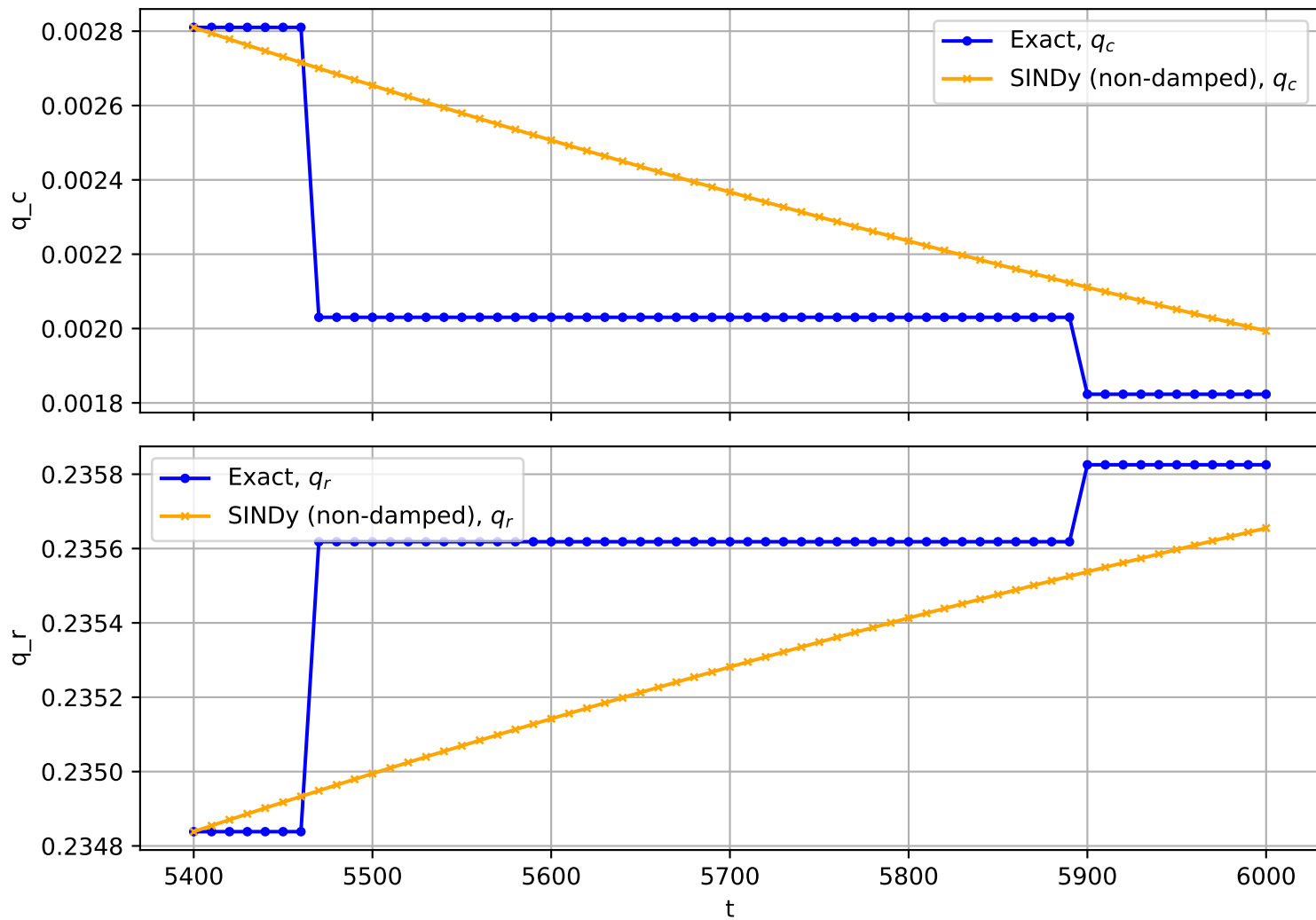
Trajectory No. 2562
