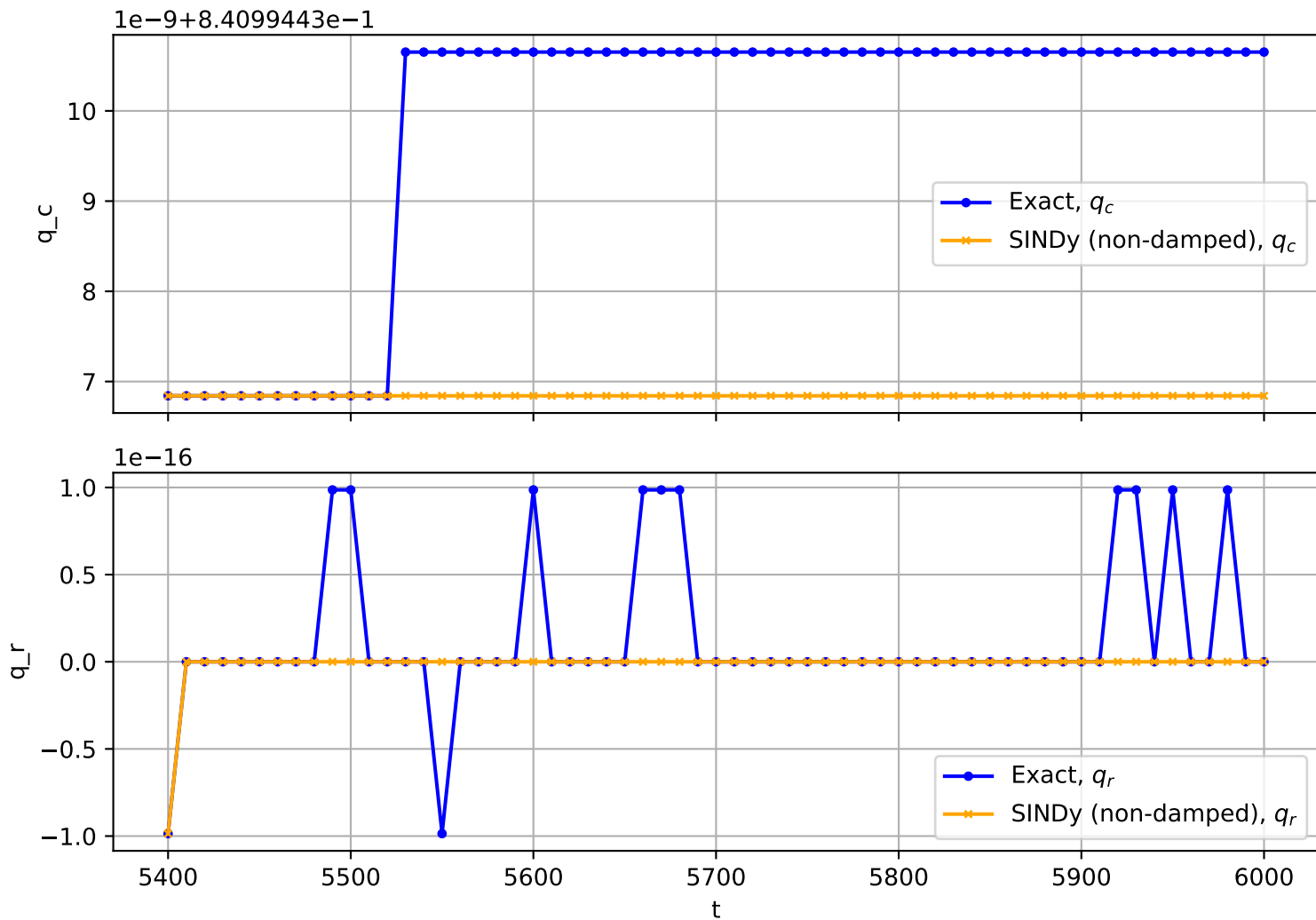
Trajectory No. 2563
