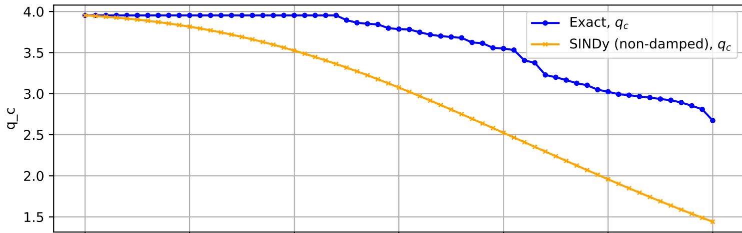
Trajectory No. 2564
