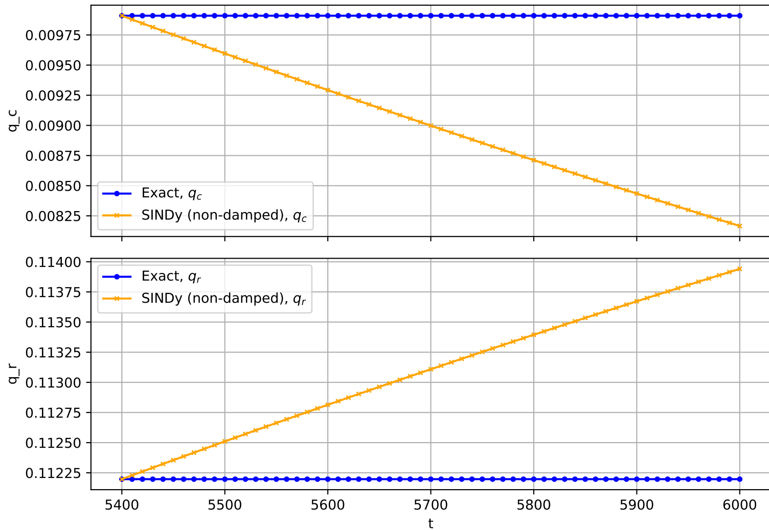
Trajectory No. 2566
