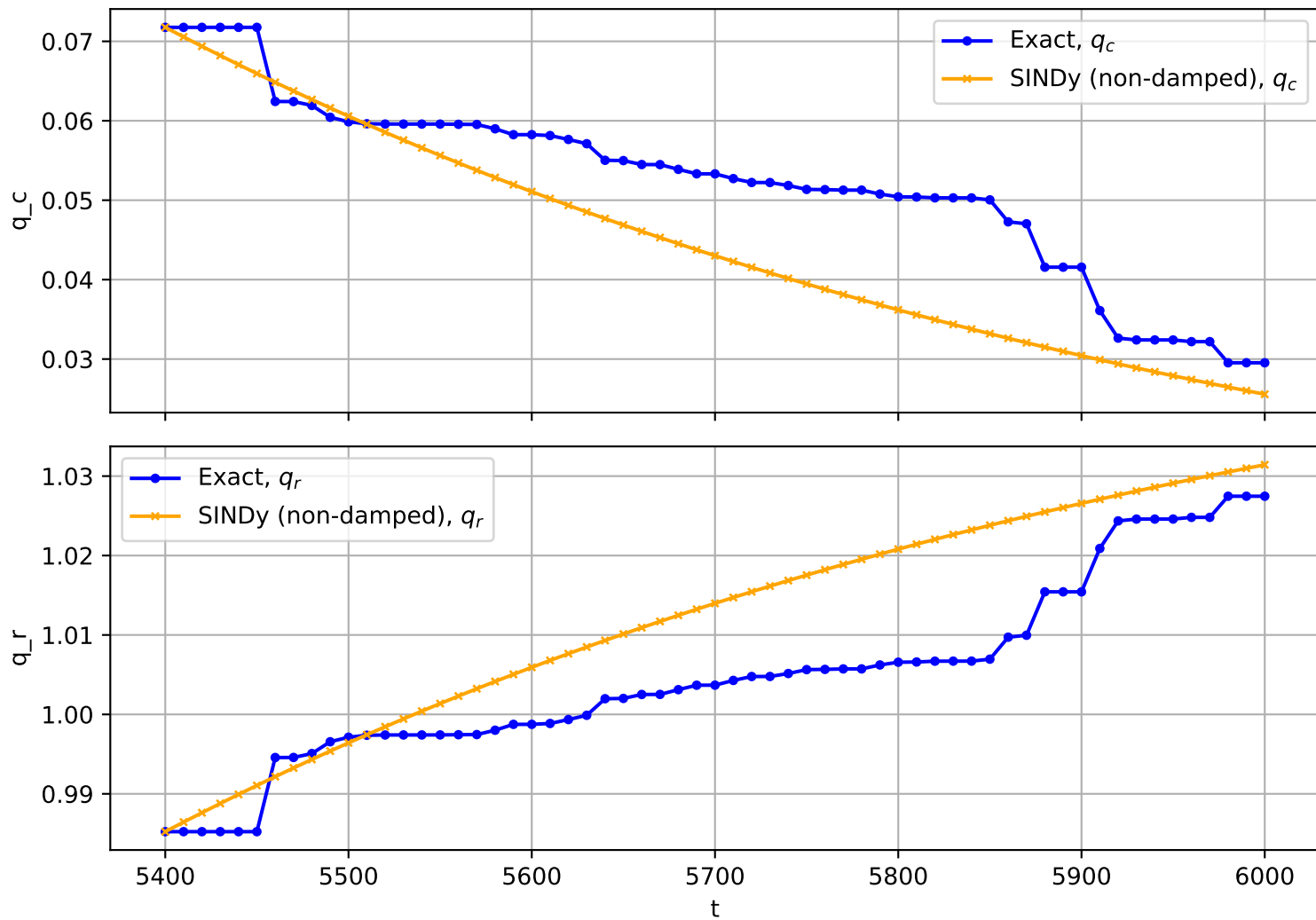
Trajectory No. 2595
