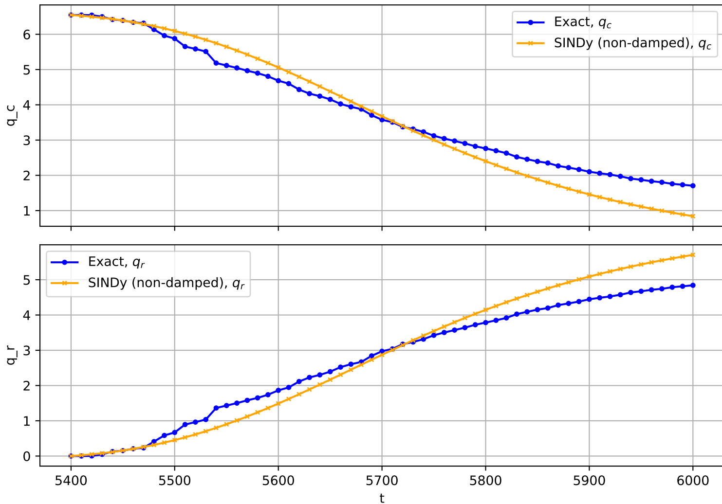
Trajectory No. 2657
