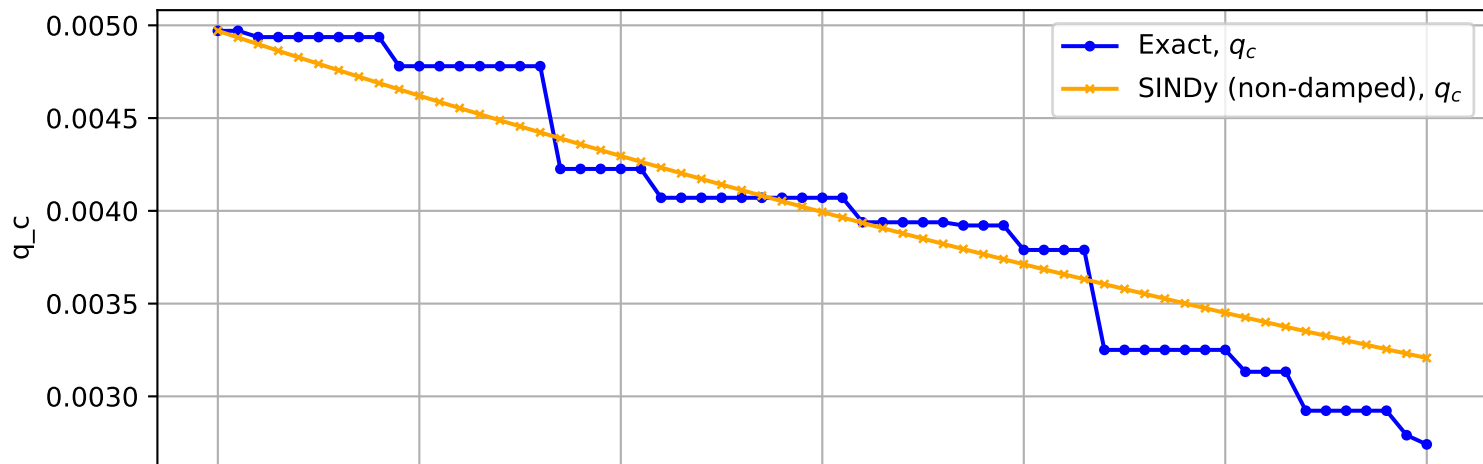
Trajectory No. 2703
