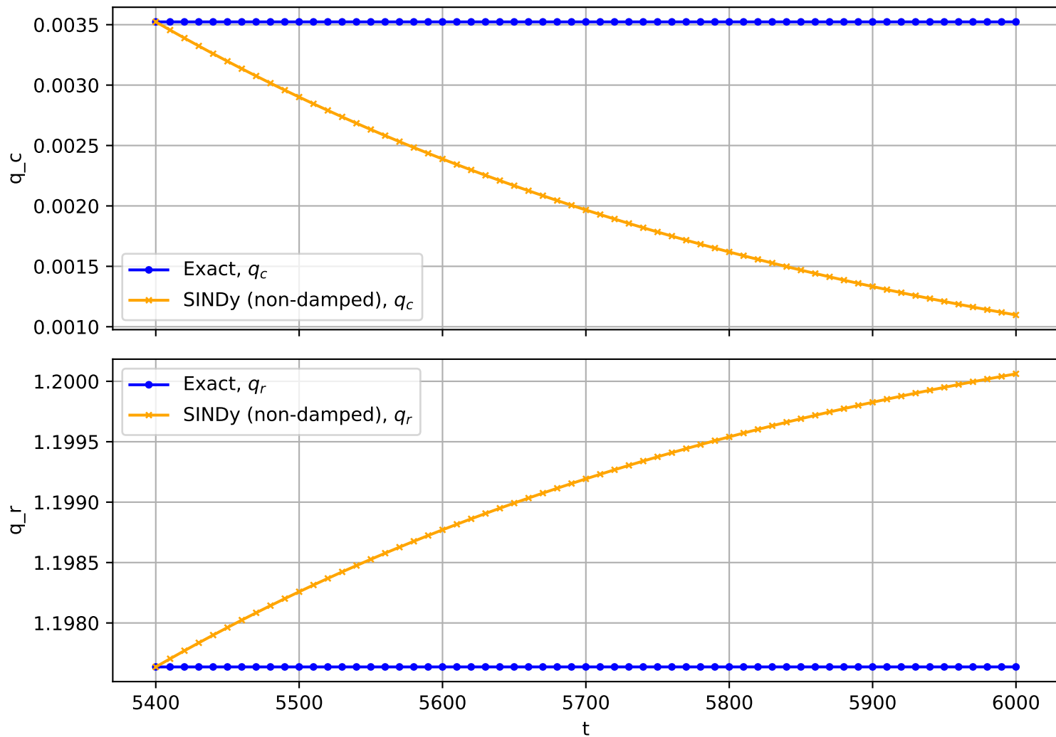
Trajectory No. 2727
