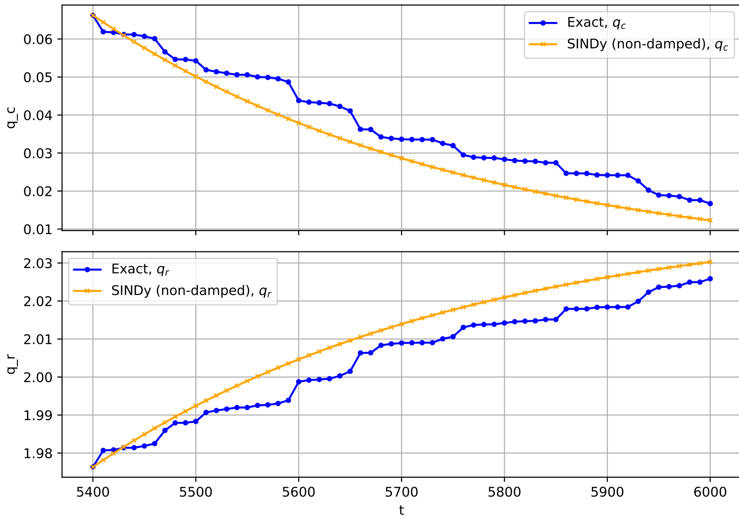
Trajectory No. 2749
