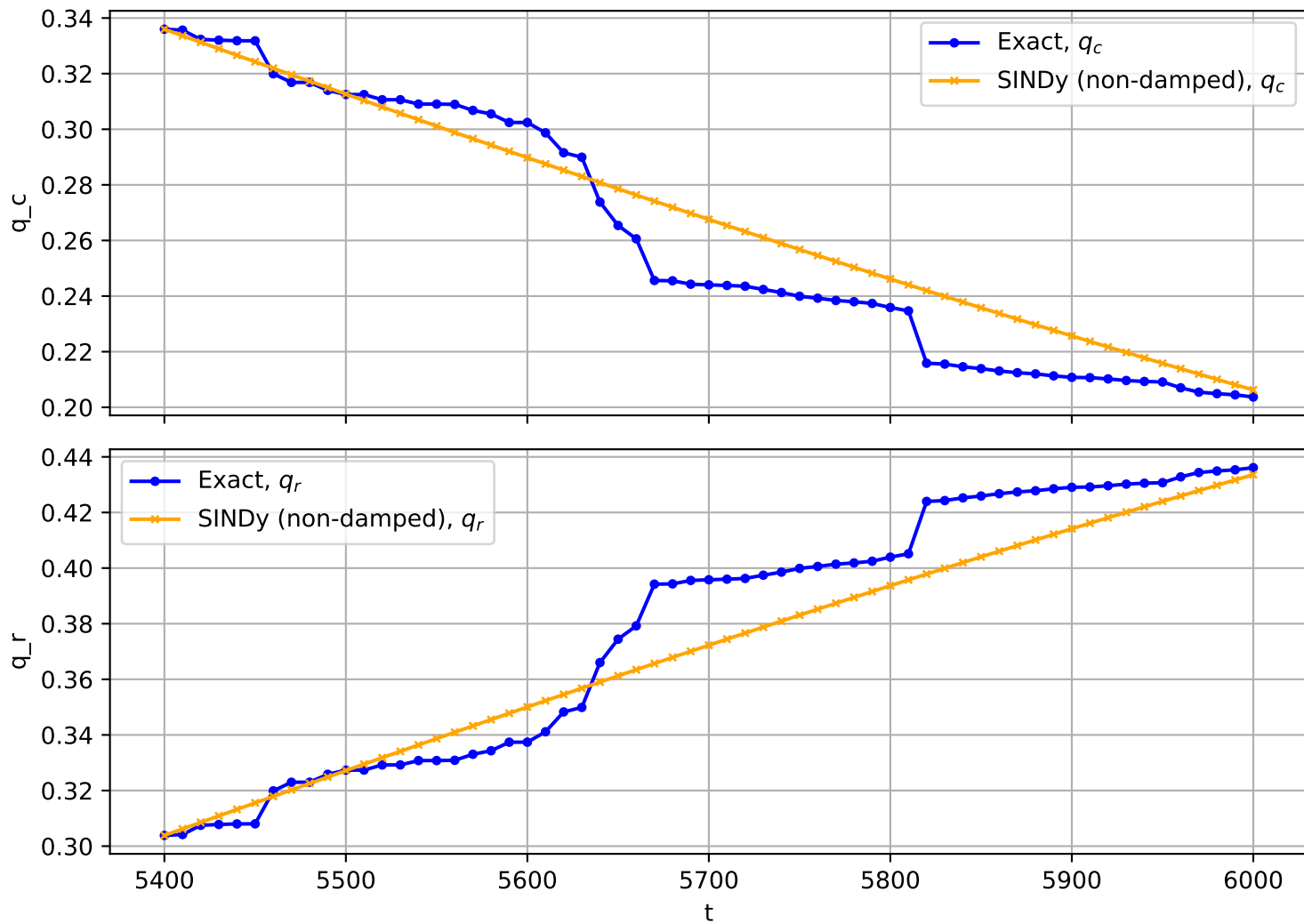
Trajectory No. 2809
