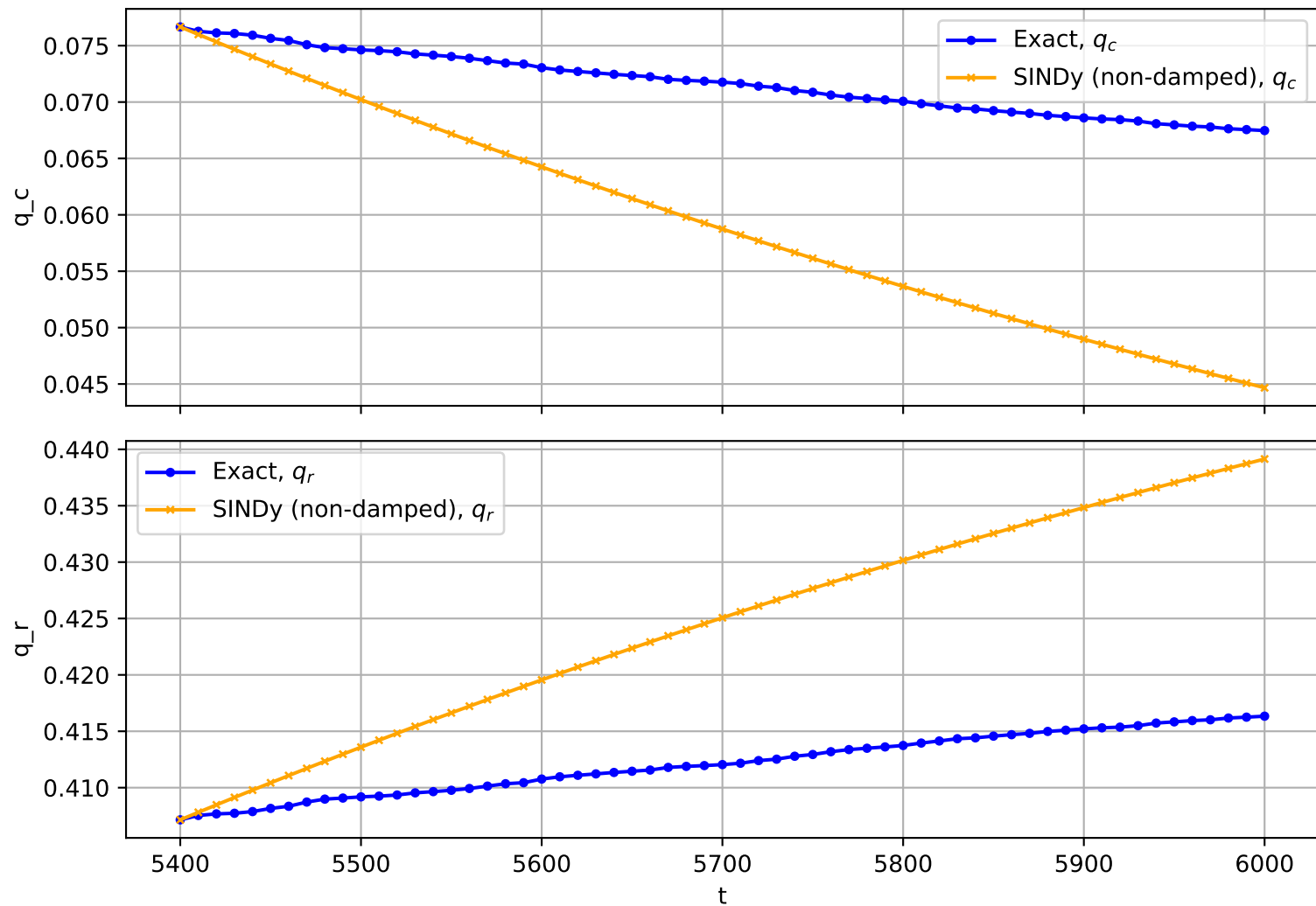
Trajectory No. 2812
