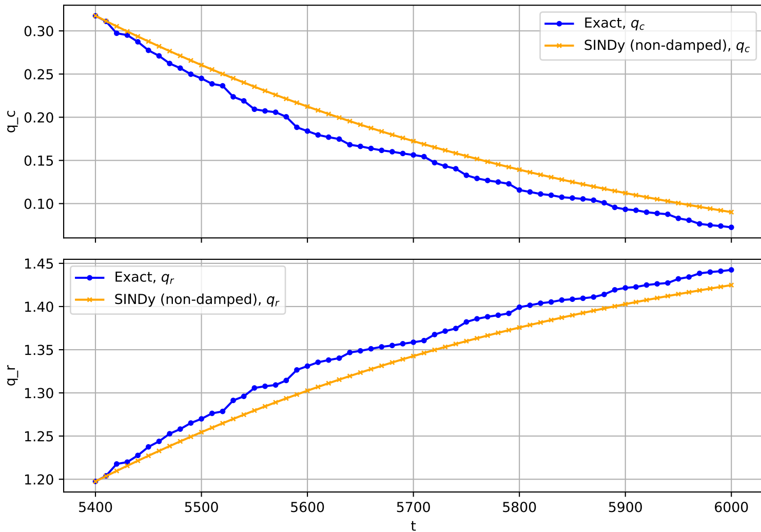
Trajectory No. 298
