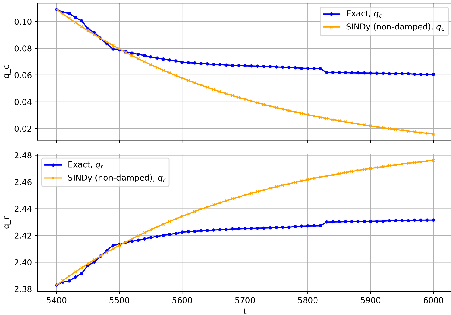
Trajectory No. 3040
