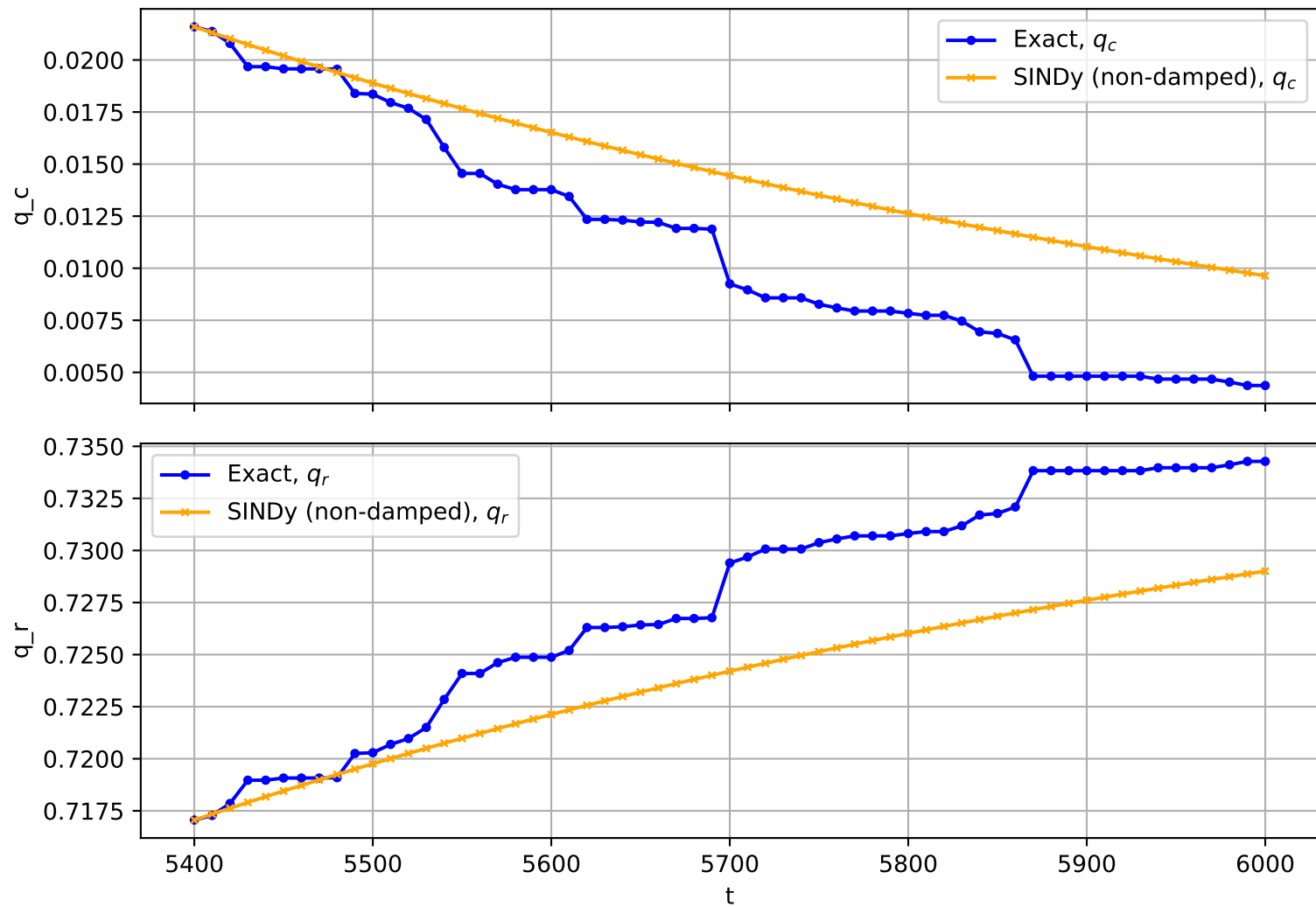
Trajectory No. 3056
