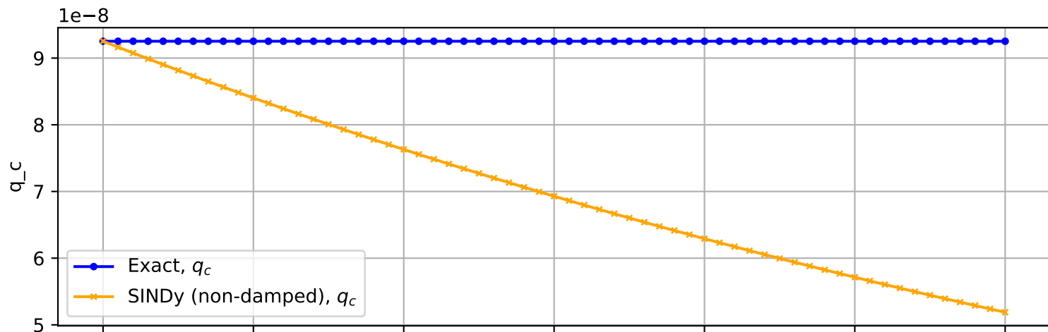
Trajectory No. 3082
