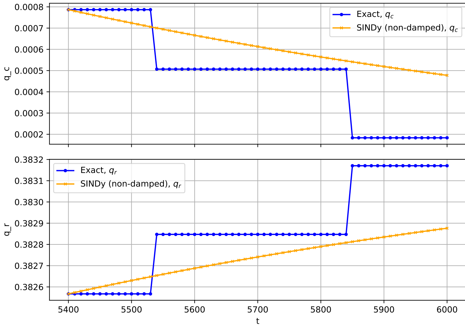
Trajectory No. 3093
