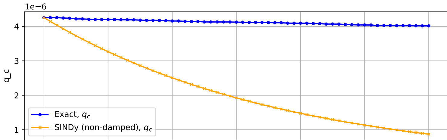
Trajectory No. 3110
