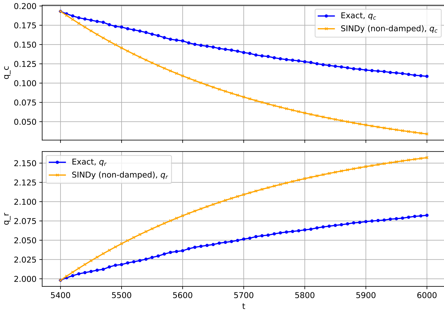
Trajectory No. 3111
