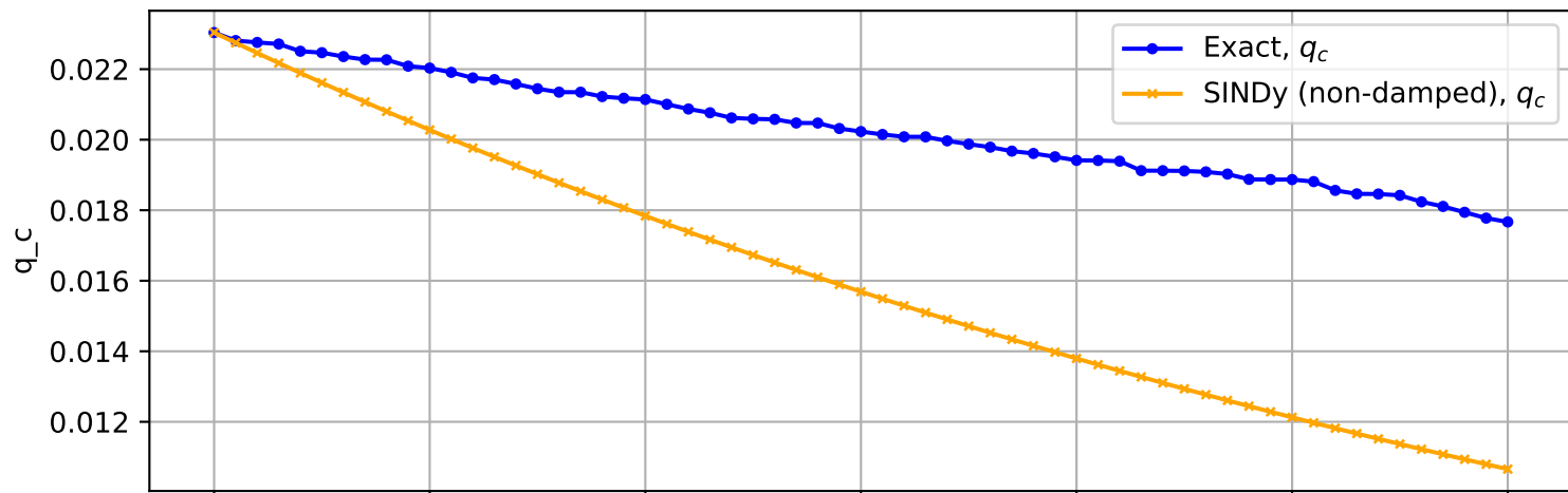
Trajectory No. 3120
