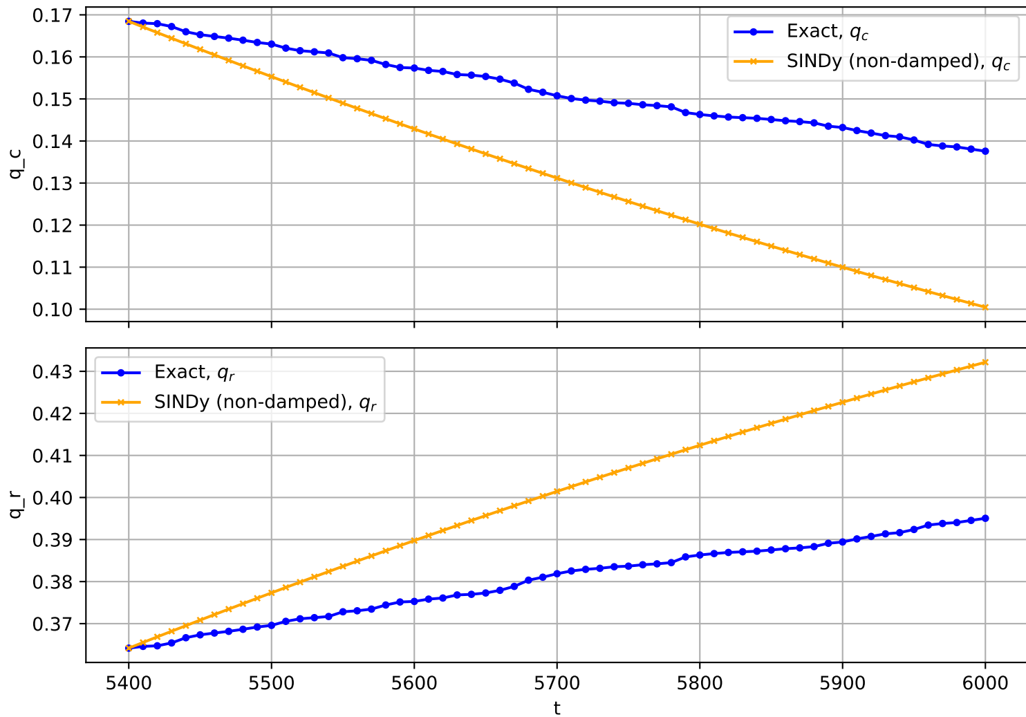
Trajectory No. 3147
