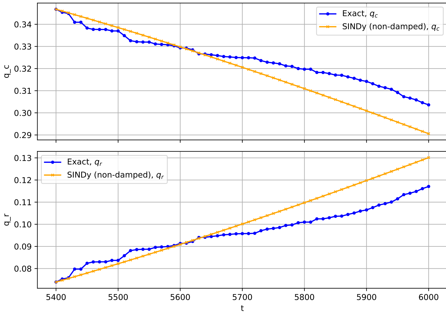
Trajectory No. 3156
