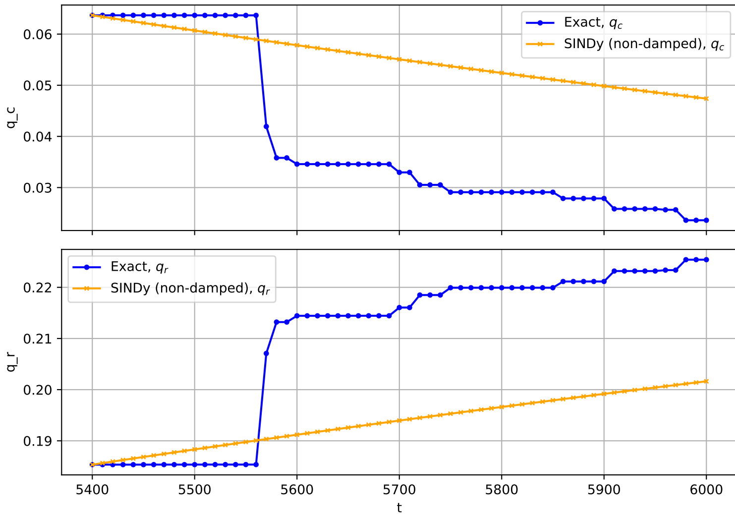
Trajectory No. 3169
