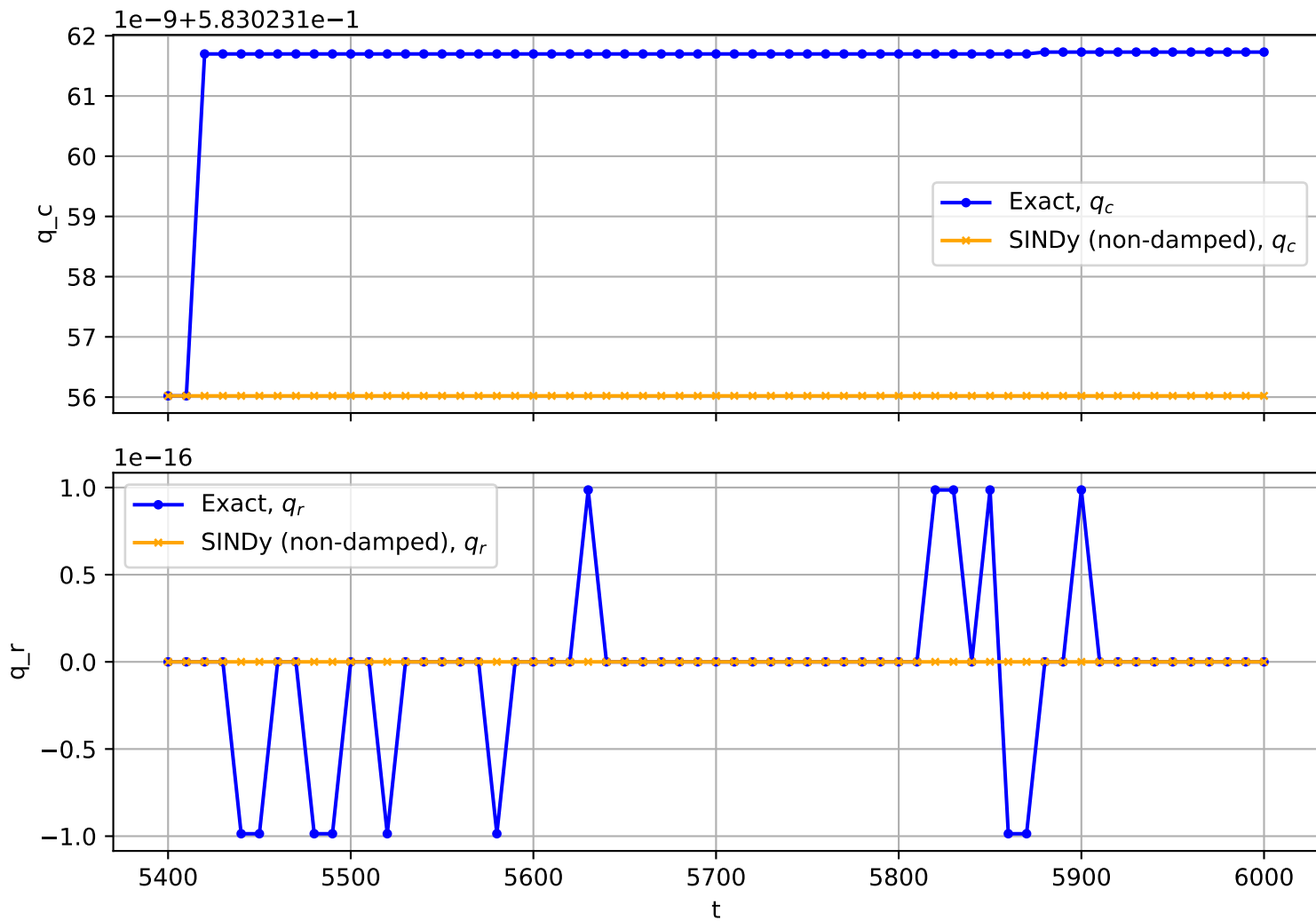
Trajectory No. 317
