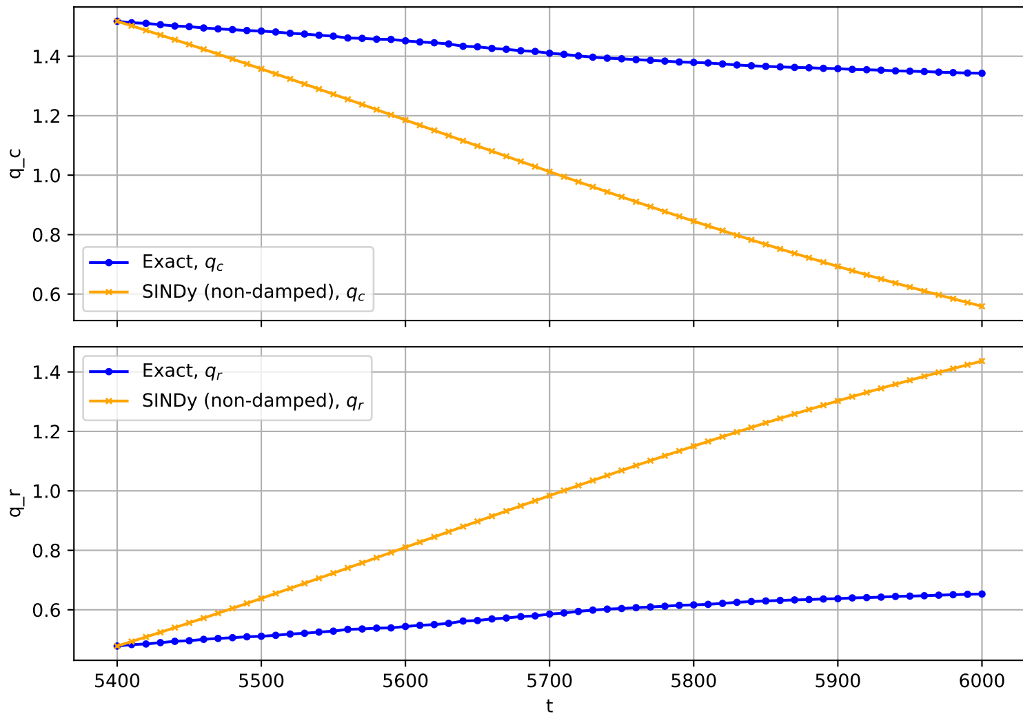
Trajectory No. 3178
