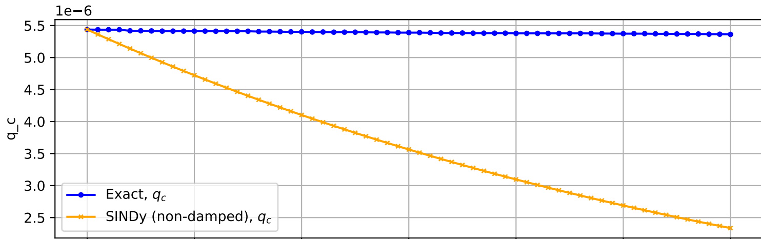
Trajectory No. 3186
