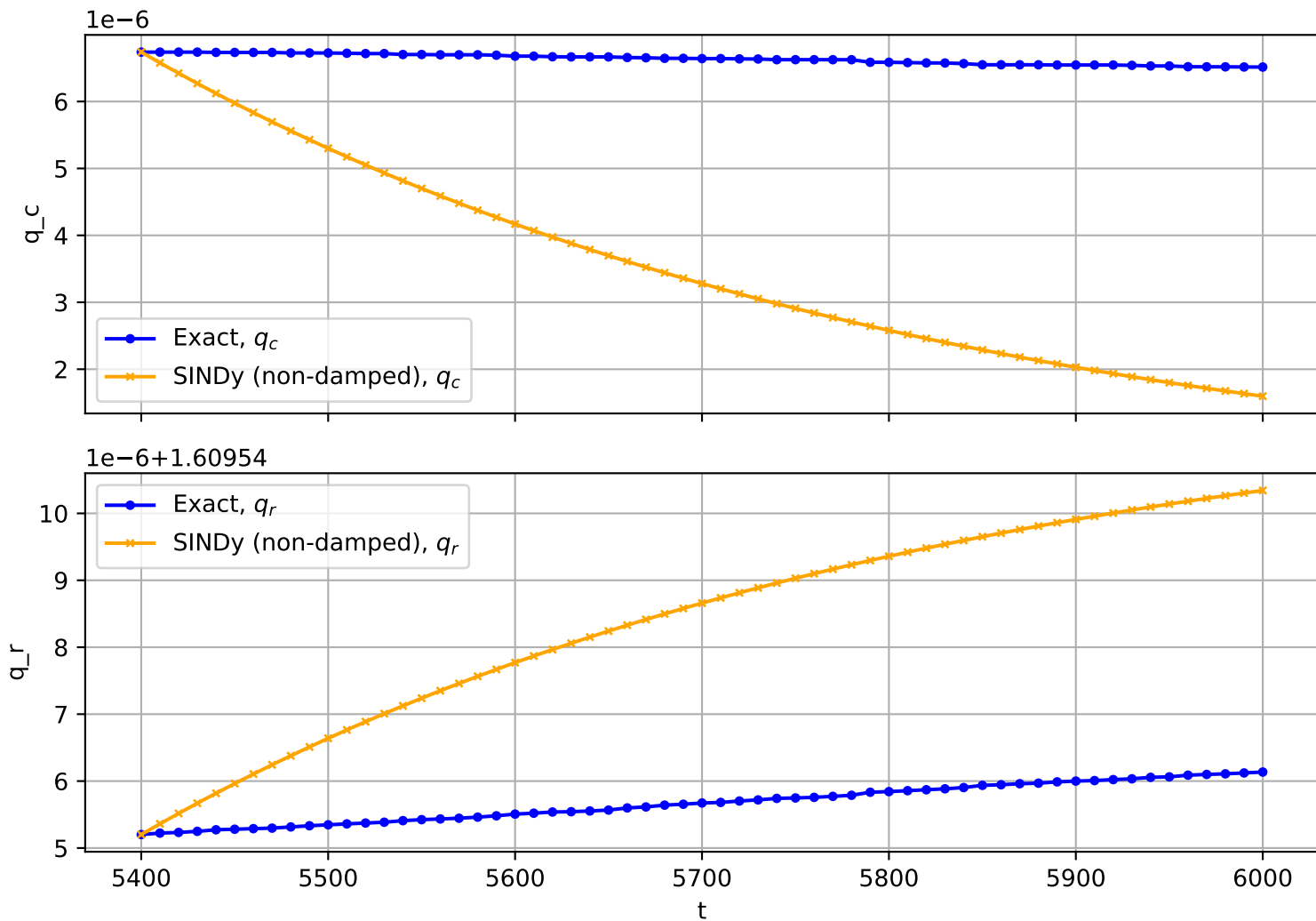
Trajectory No. 3204
