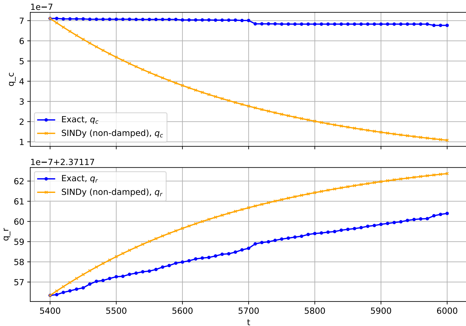
Trajectory No. 3210
