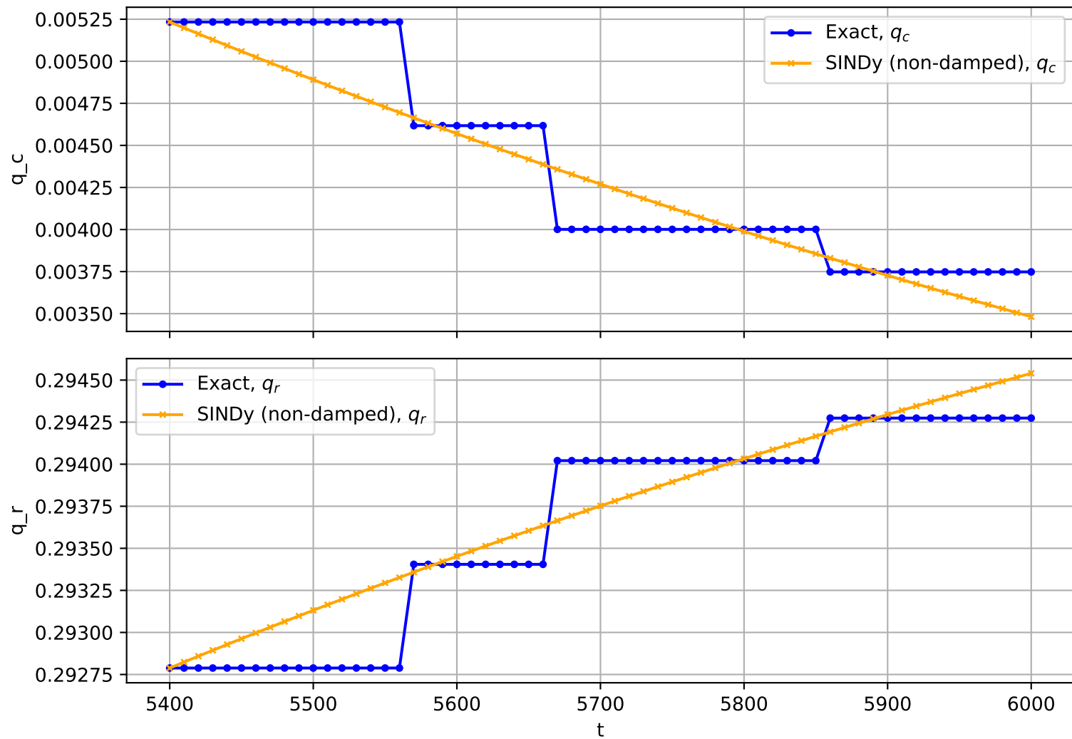
Trajectory No. 3230
