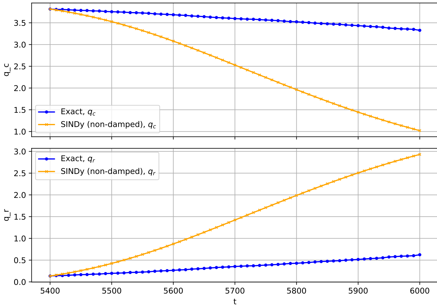
Trajectory No. 3257
