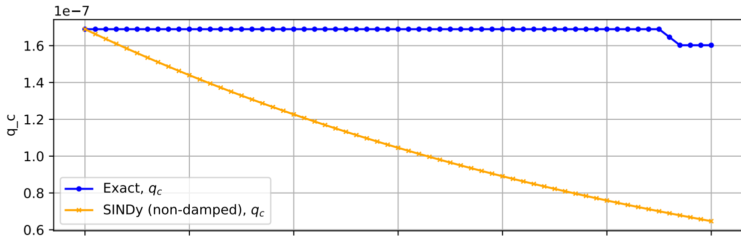
Trajectory No. 3284
