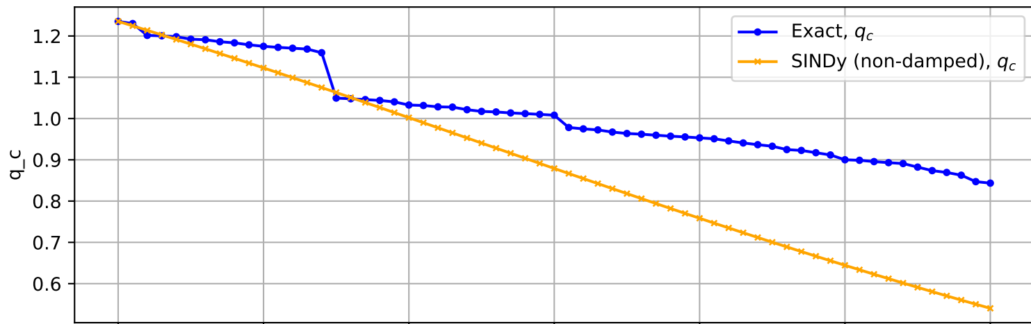
Trajectory No. 3296
