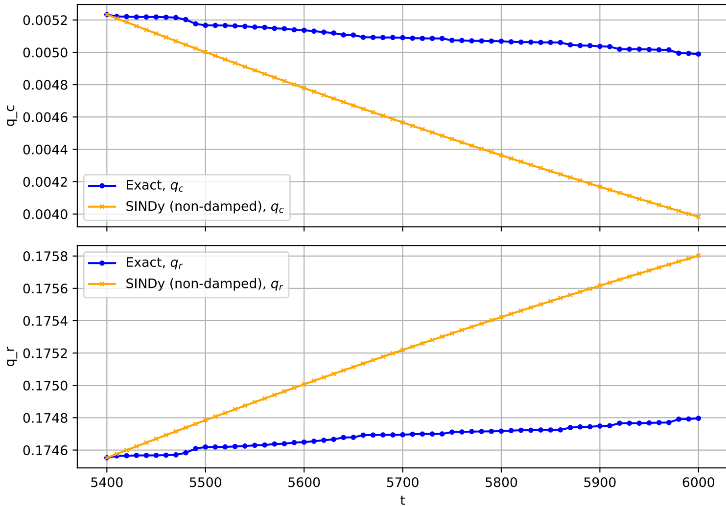
Trajectory No. 3300
