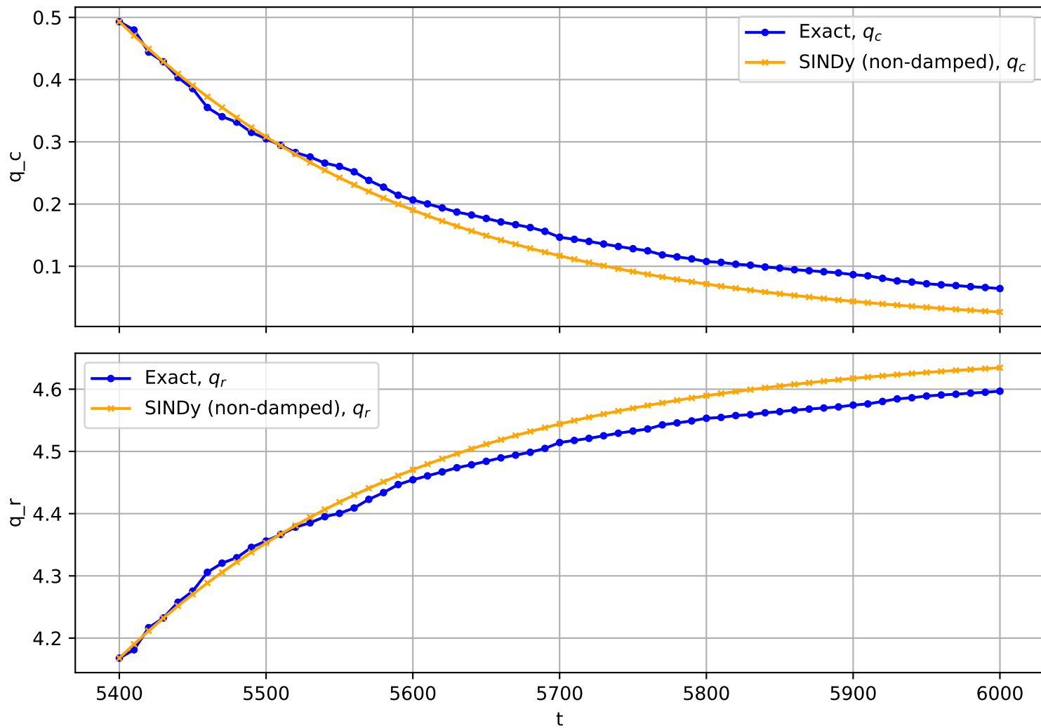
Trajectory No. 3303
