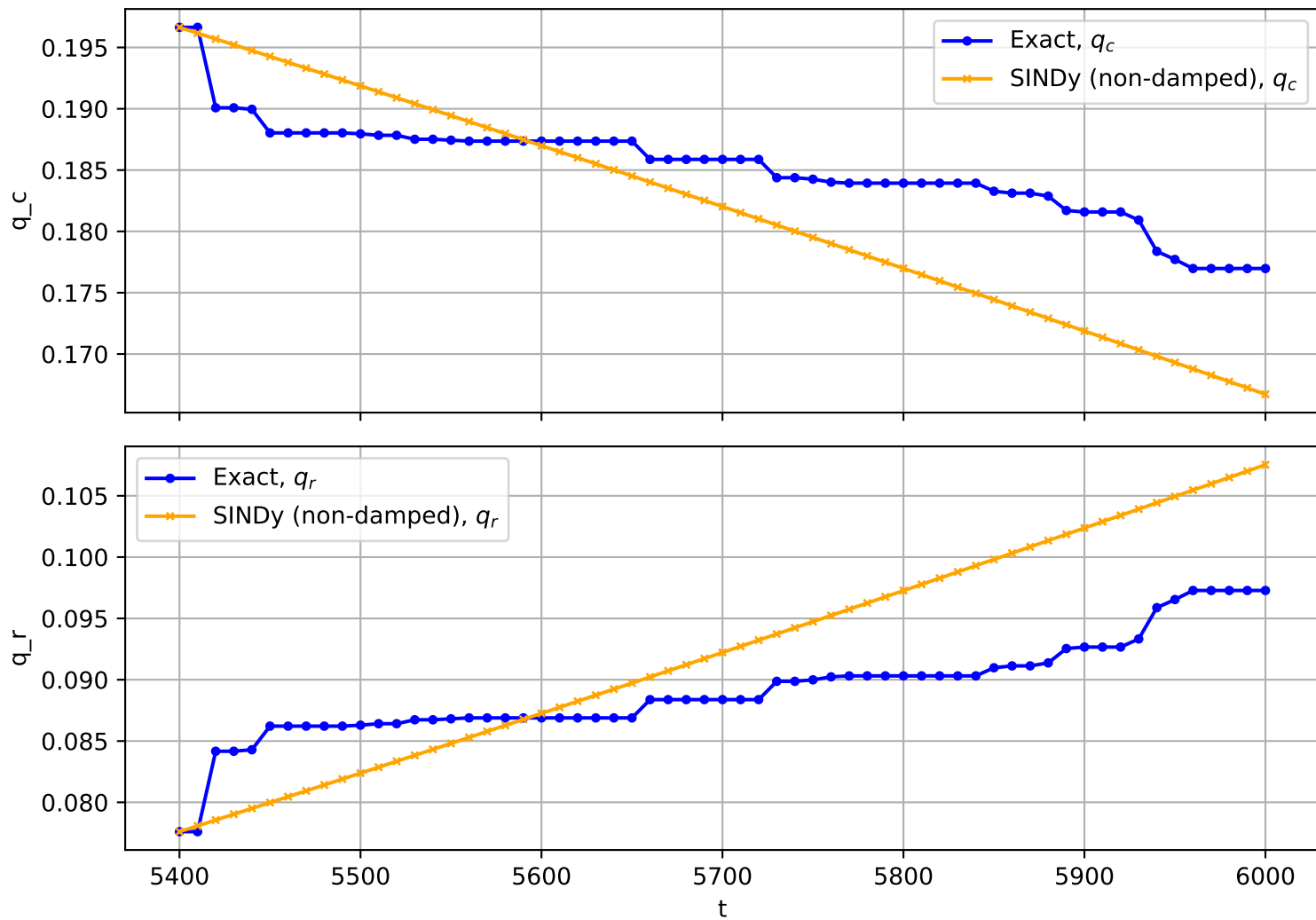
Trajectory No. 3316
