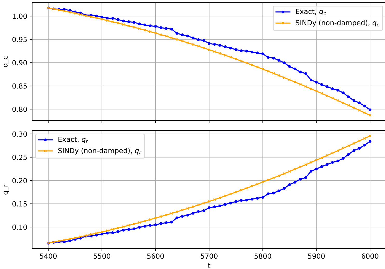
Trajectory No. 3344
