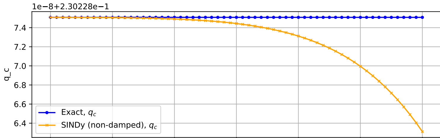
Trajectory No. 3350
