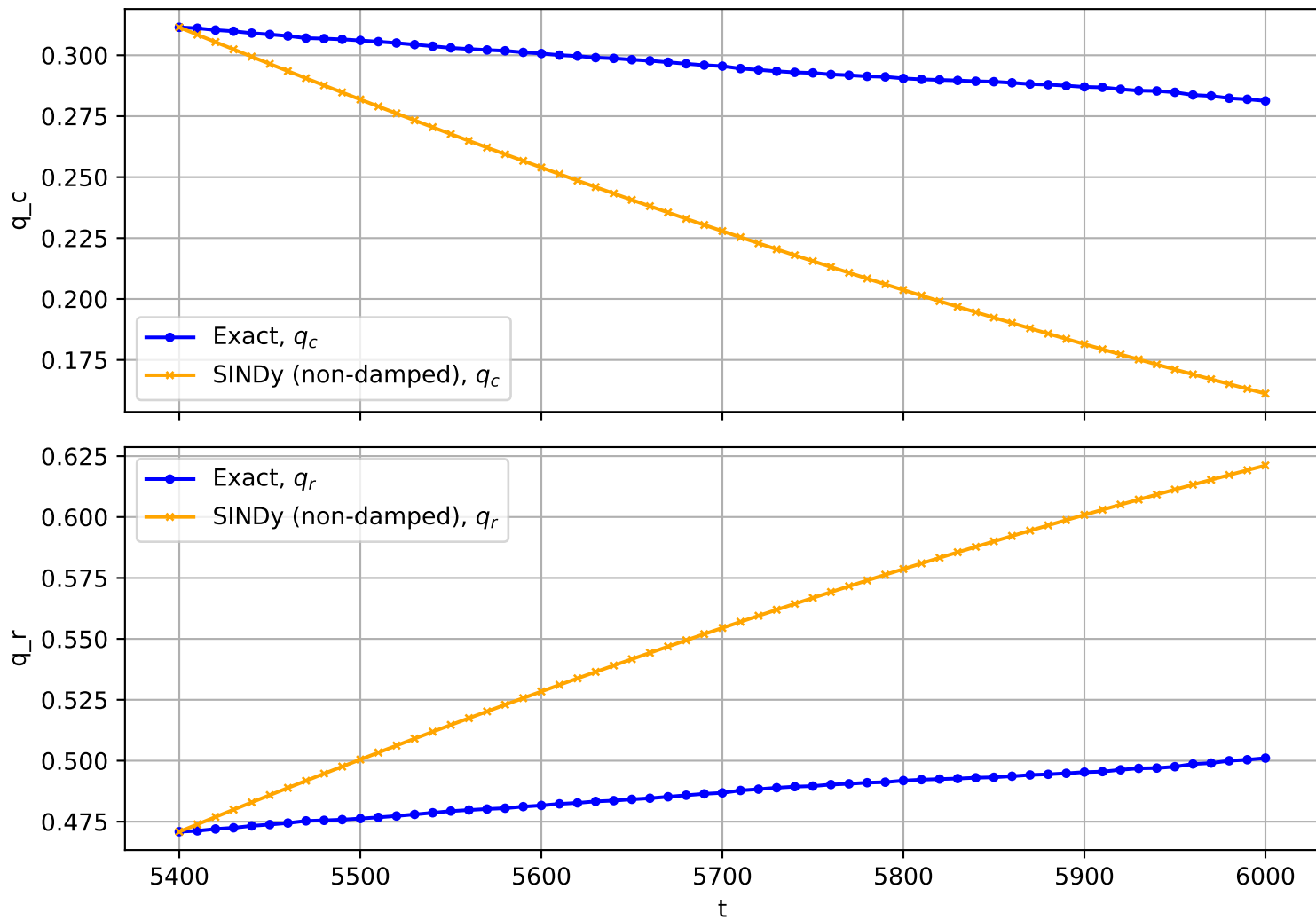
Trajectory No. 3354
