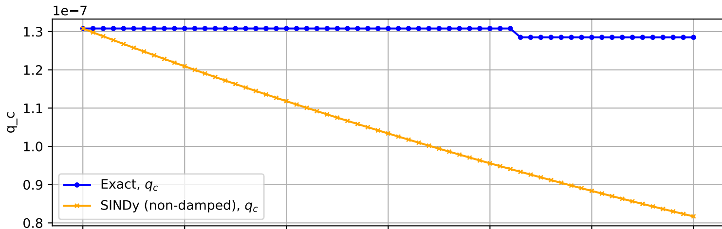
Trajectory No. 3359
