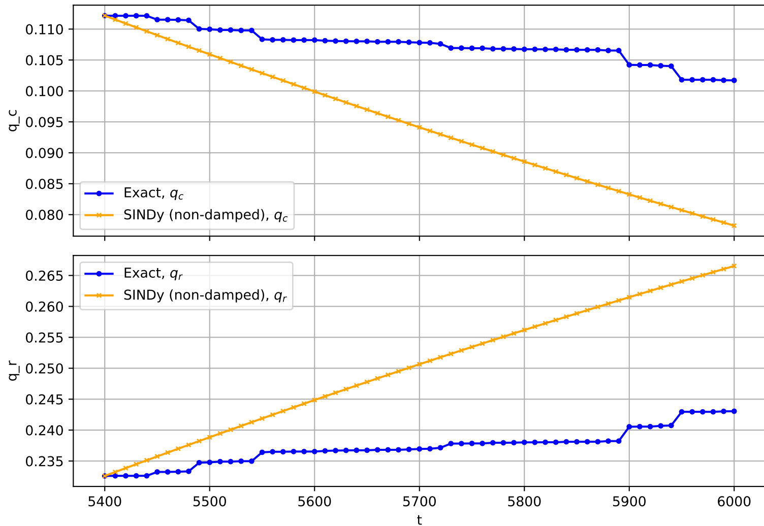
Trajectory No. 3378
