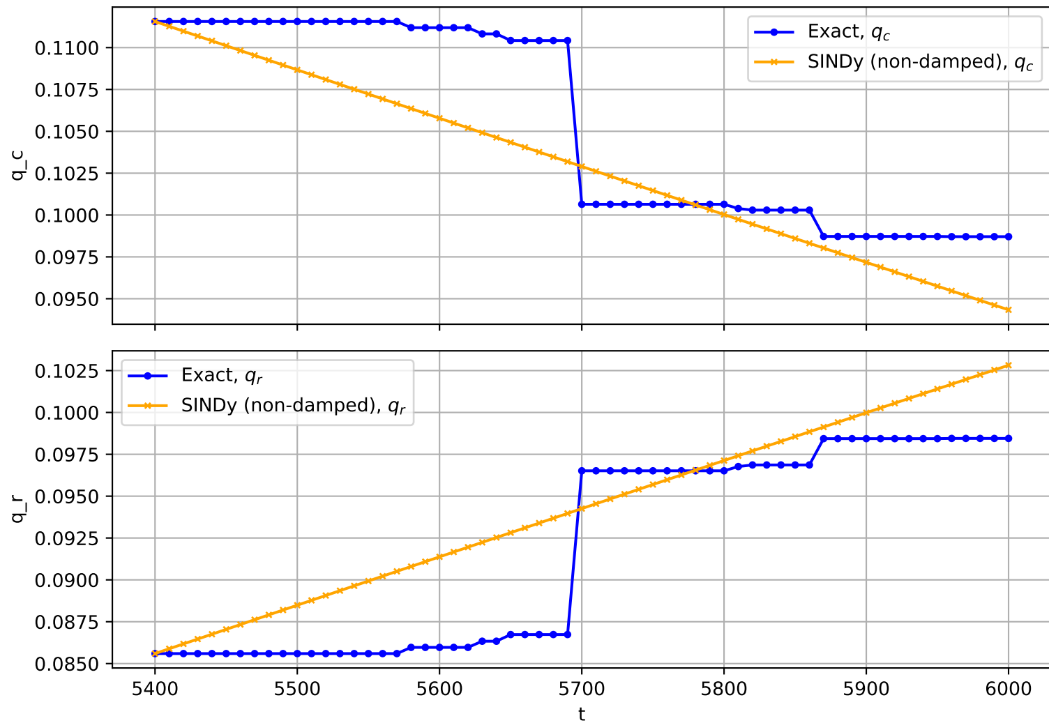
Trajectory No. 3379
