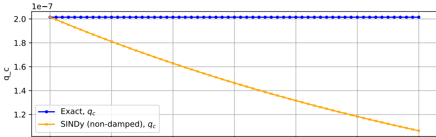
Trajectory No. 3385
