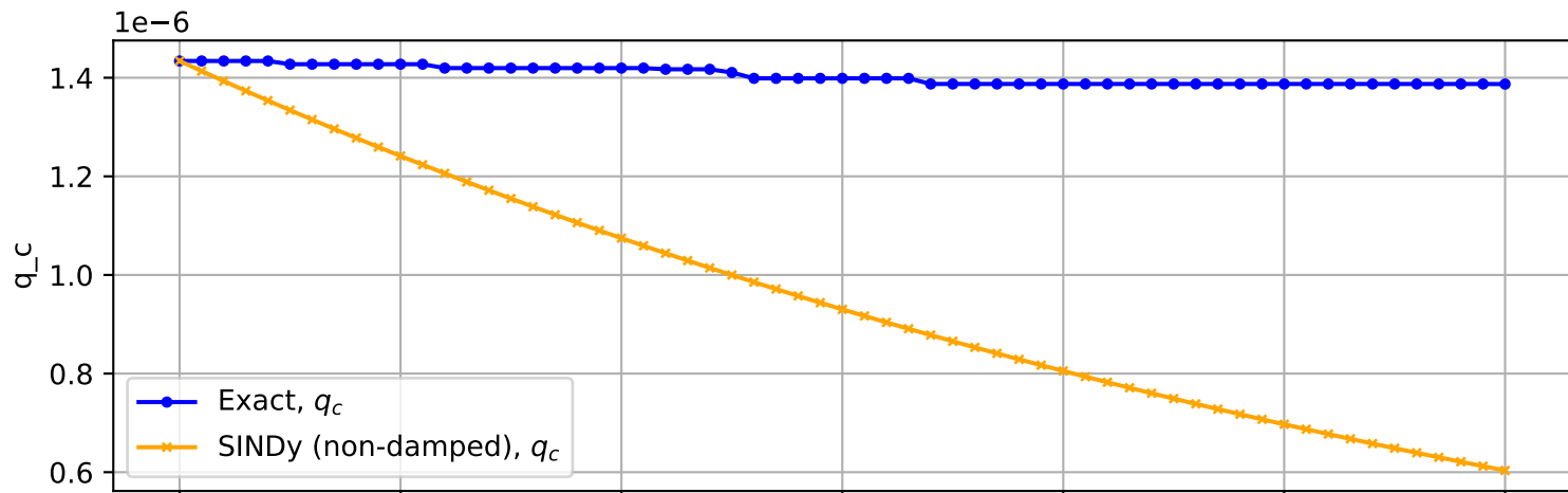
Trajectory No. 3387
