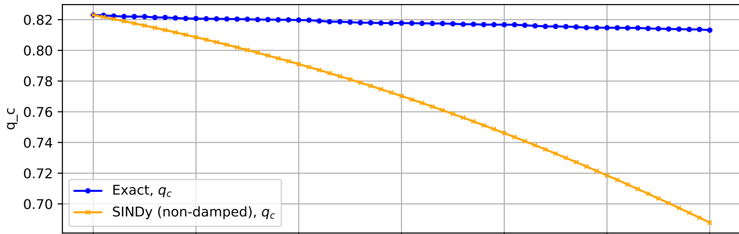
Trajectory No. 3413
