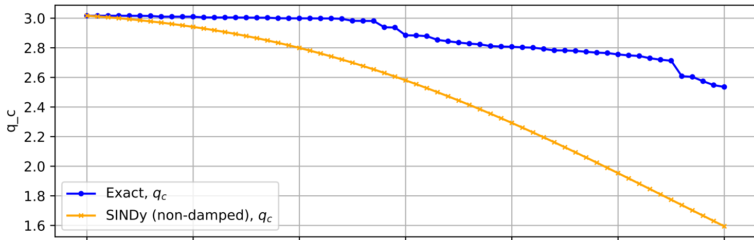
Trajectory No. 3422
